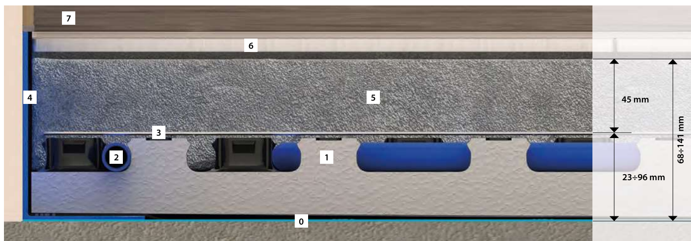
Pannello Kilma-Strong Serie 1188
